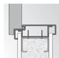
zárubeň Rohová VELKÁ montáž na stěně SDK
